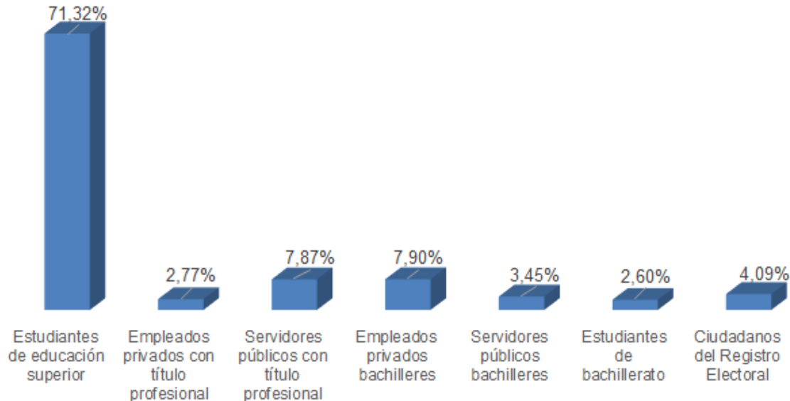
Figura 6. Estadísticas sobre la selección de MJRV
